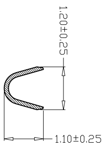
SECTION A-A SCALE 1:1
